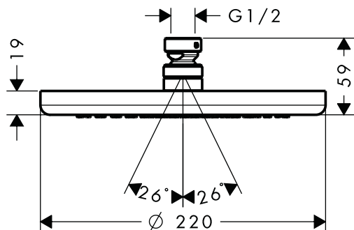
Croma 220 26464000
