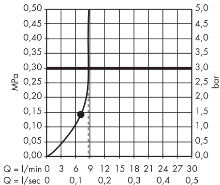
Croma 220 26465000
