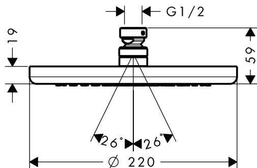
Croma 220 26465000
