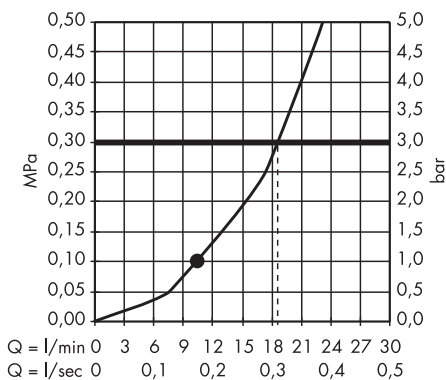
Croma 220 26464000
